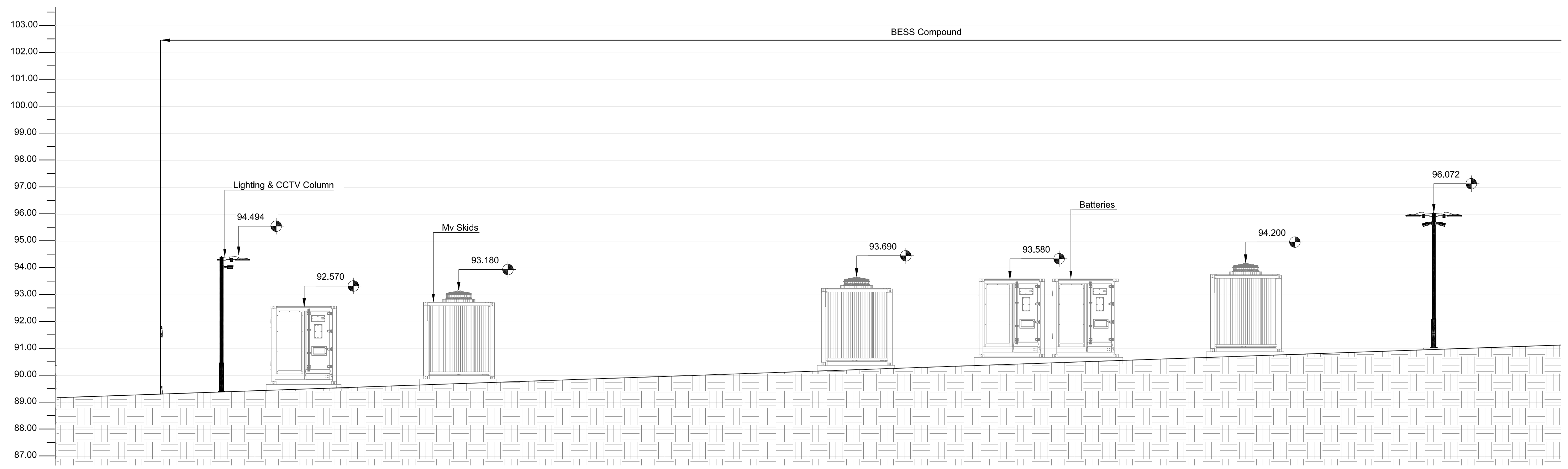
13 SECTION F - F Scale: 1:100
