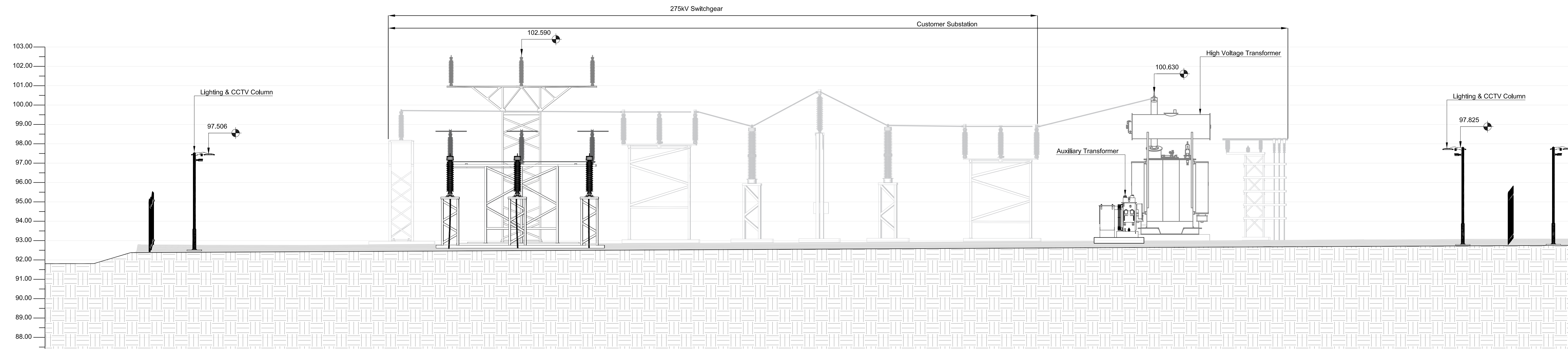
2 SECTION A - A Scale: 1:100(B/A)
