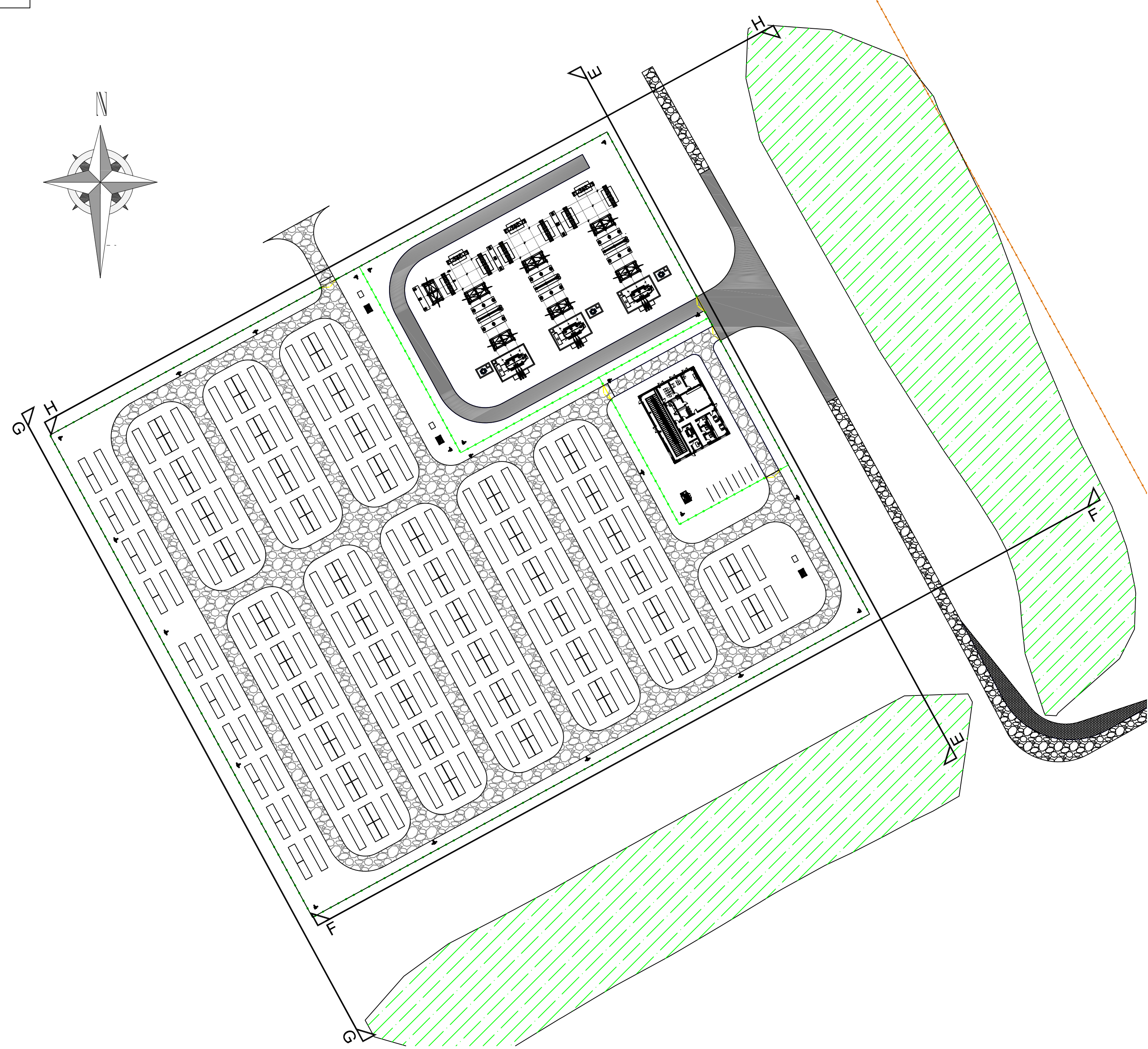
12 KEY PLAN 2 Scale: 1:1000
